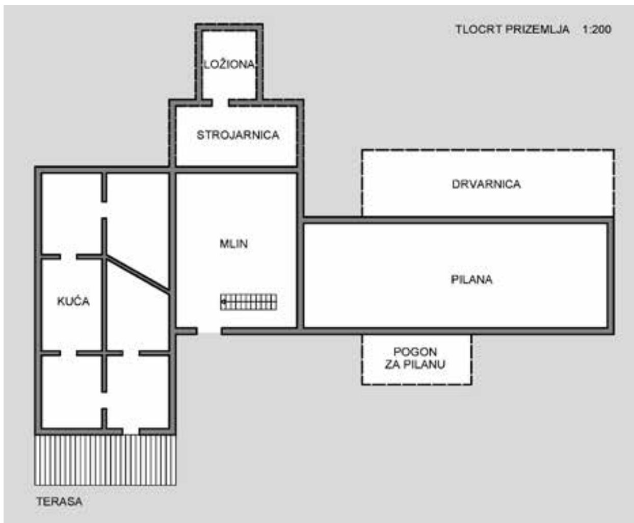
Tlocrt mlina izradio Jonatan Berlančić na temelju skice Petra Radenovića
